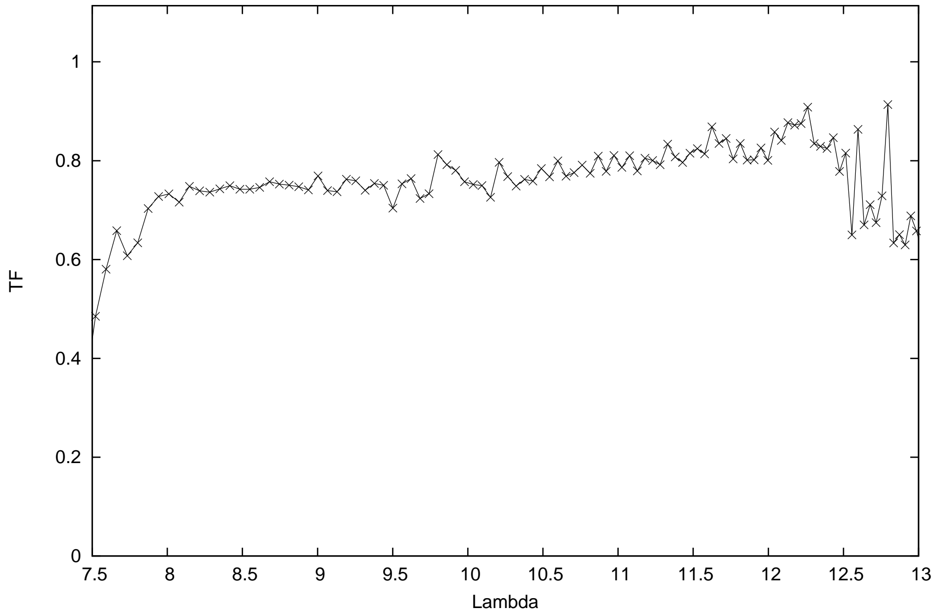
calHD81797_flux-1.49_diam9.14_r.MIDI.2015-03-05T04_17_52.000_G111
