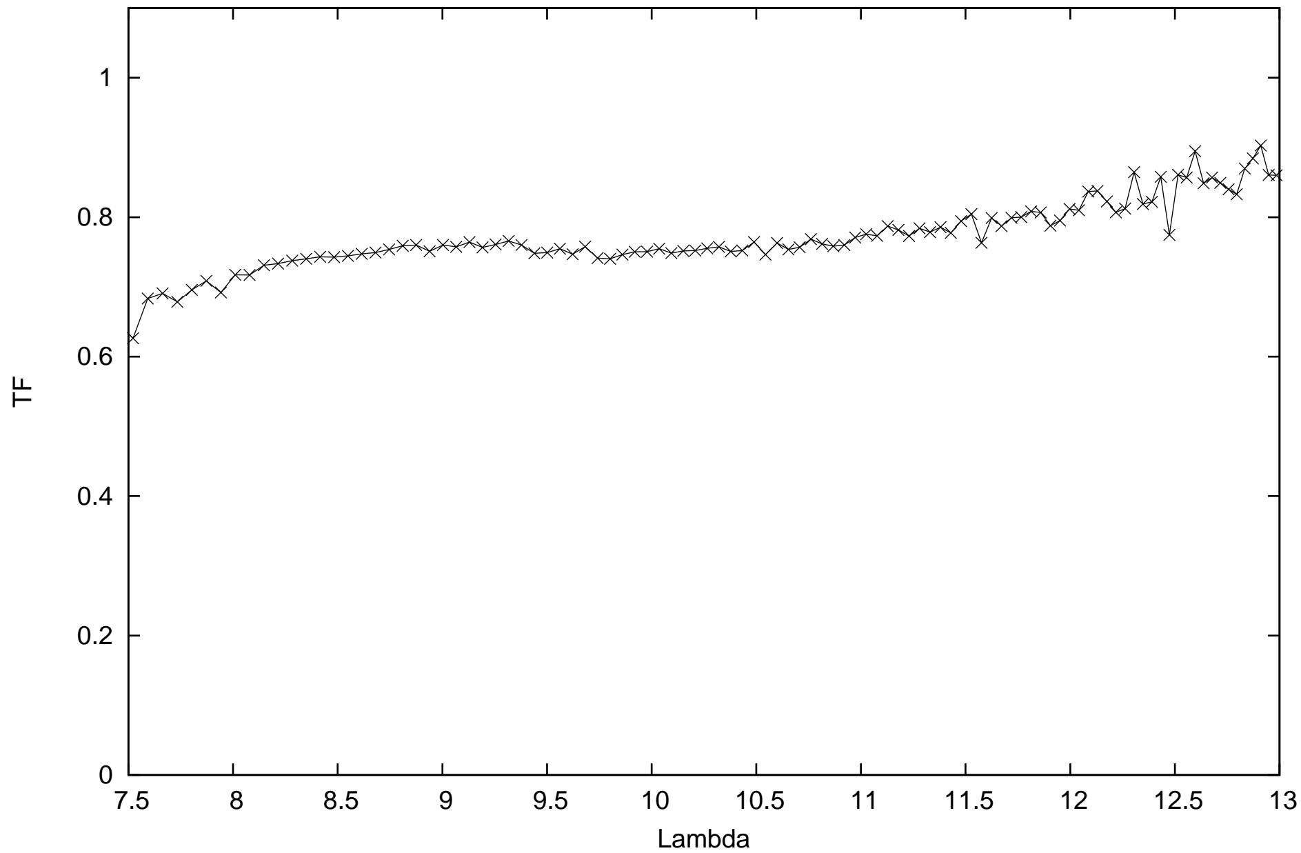
calHD81797_flux-1.49_diam9.14_r.MIDI.2015-03-05T03_35_30.000_G111
