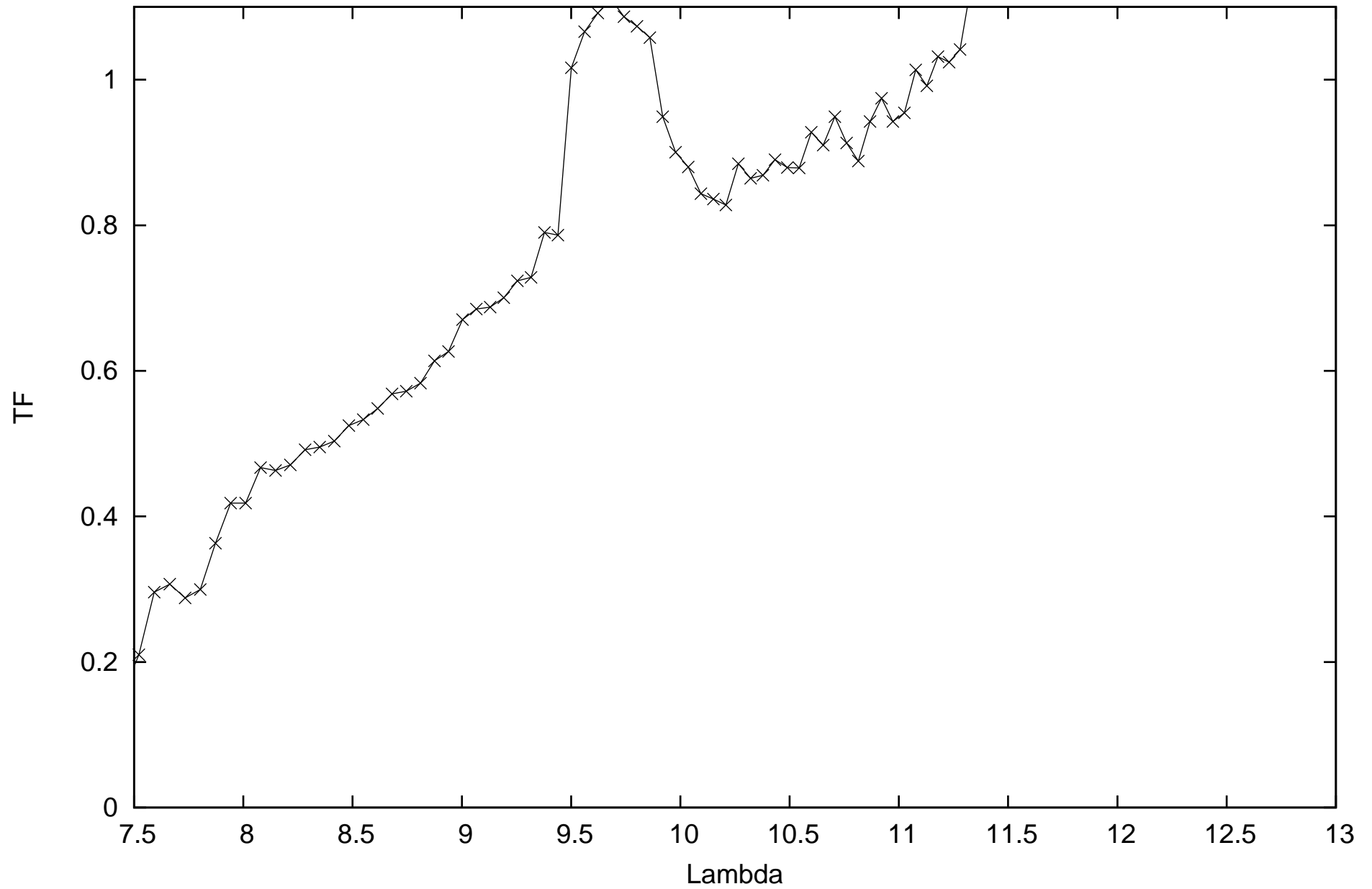
calHIP98337_flux-0.45181_diam5.93_r.MIDI.2014-06-01T08_27_50.000_A111
