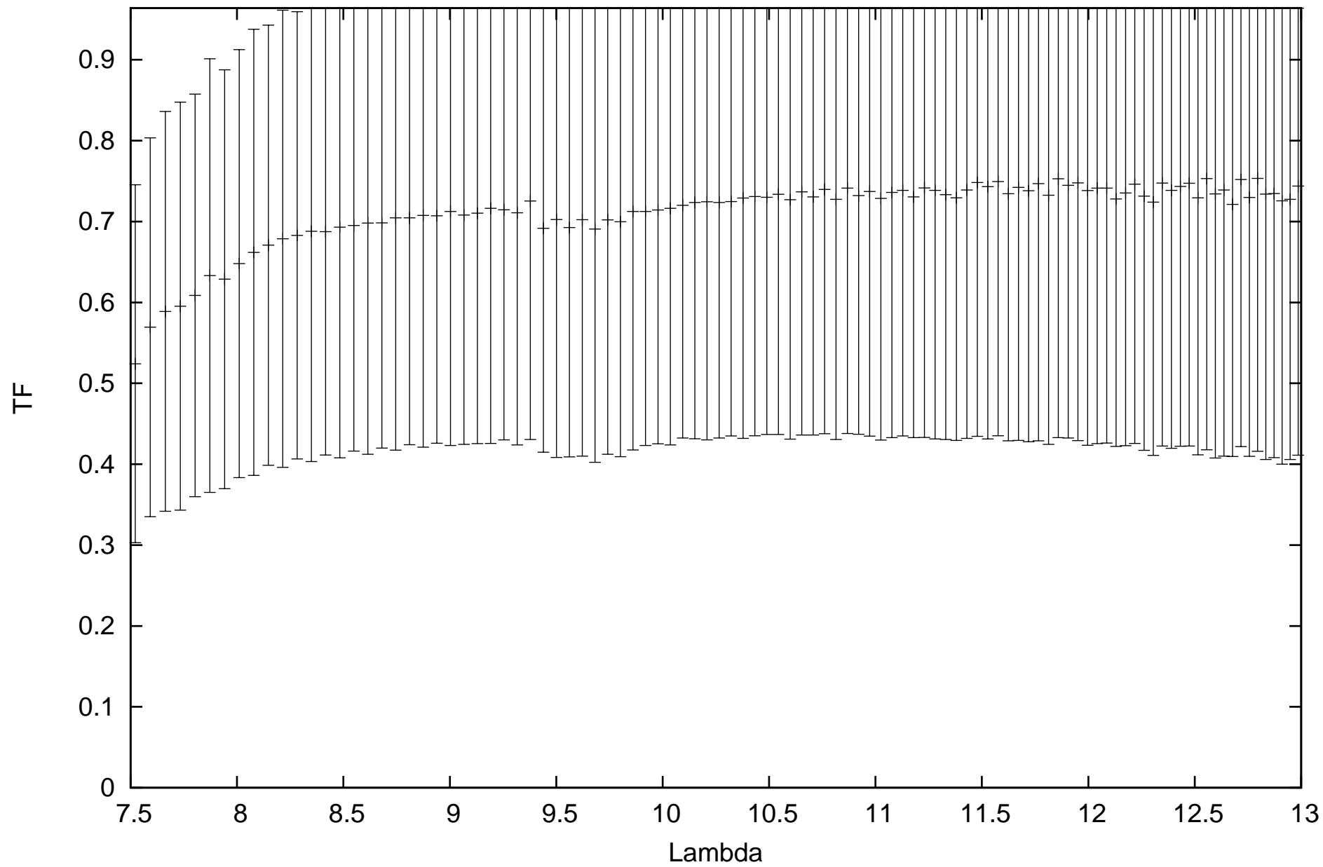
calHIP13701_flux1.17204_diam2.55_r.MIDI.2014-11-04T05_21_24.000_U3U4
