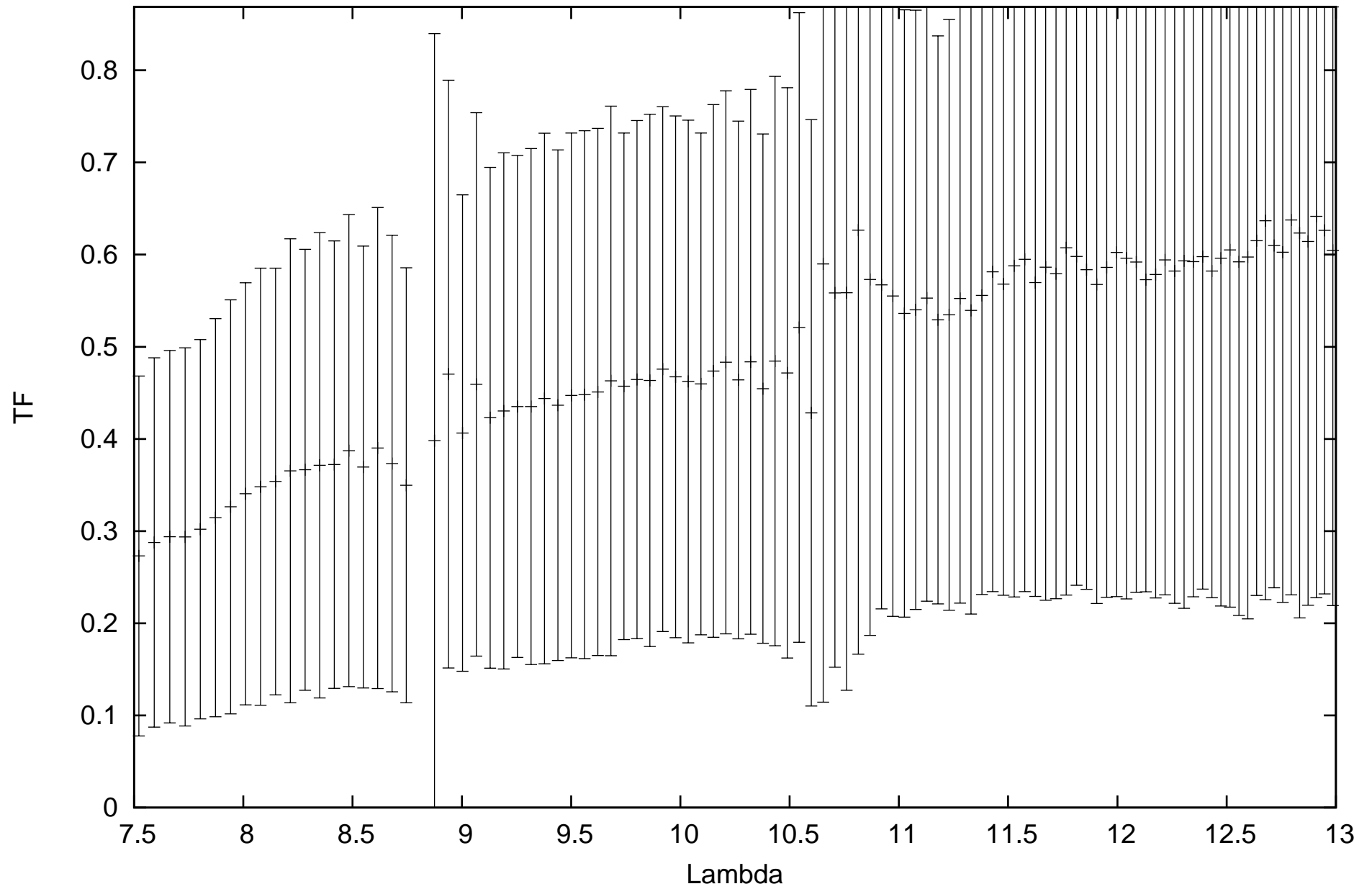
calHD167618_flux-1.82_diam11.66_r.MIDI.2014-07-07T03_18_15.000_C1A1
