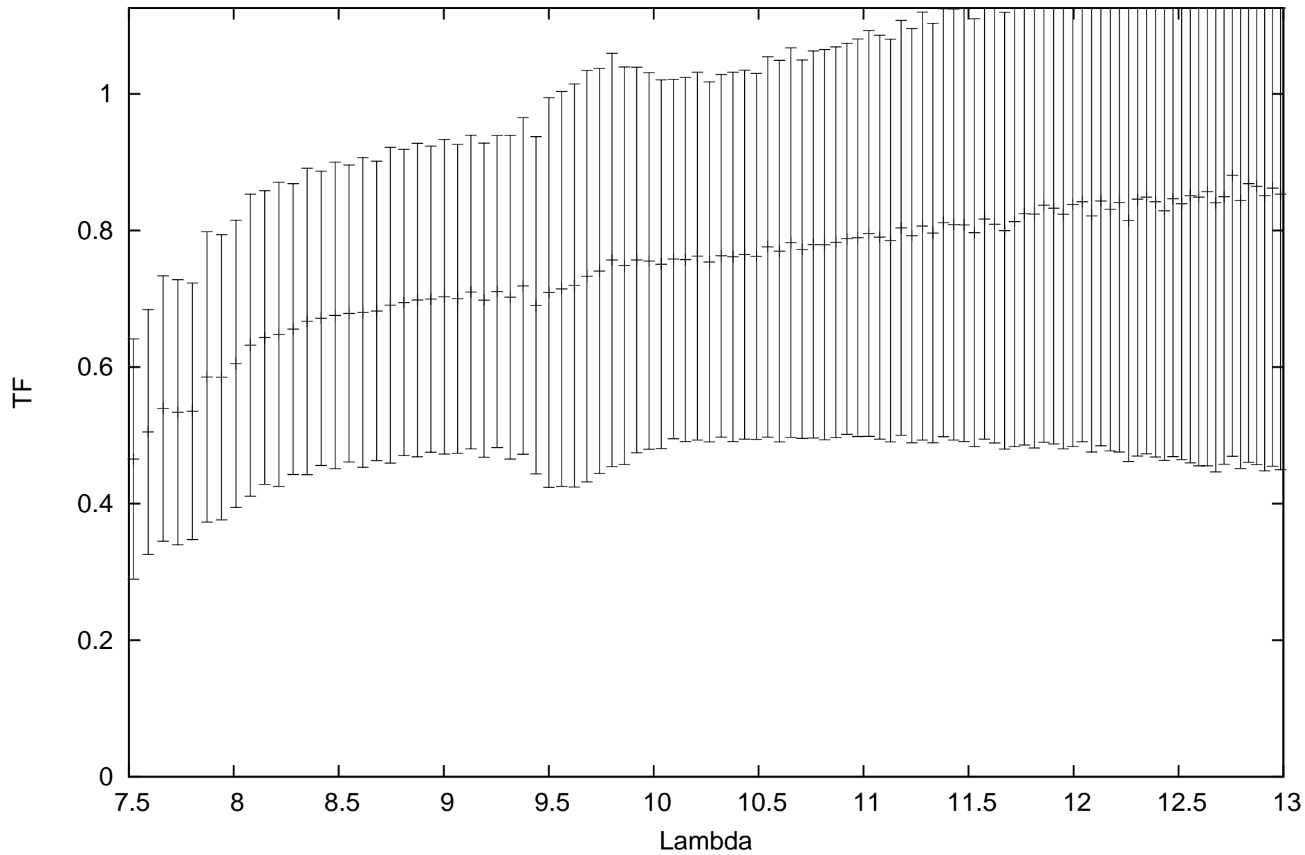
calHD151011_flux1.28_diam2.85_r.MIDI.2014-04-16T09_14_04.000_U3U4
