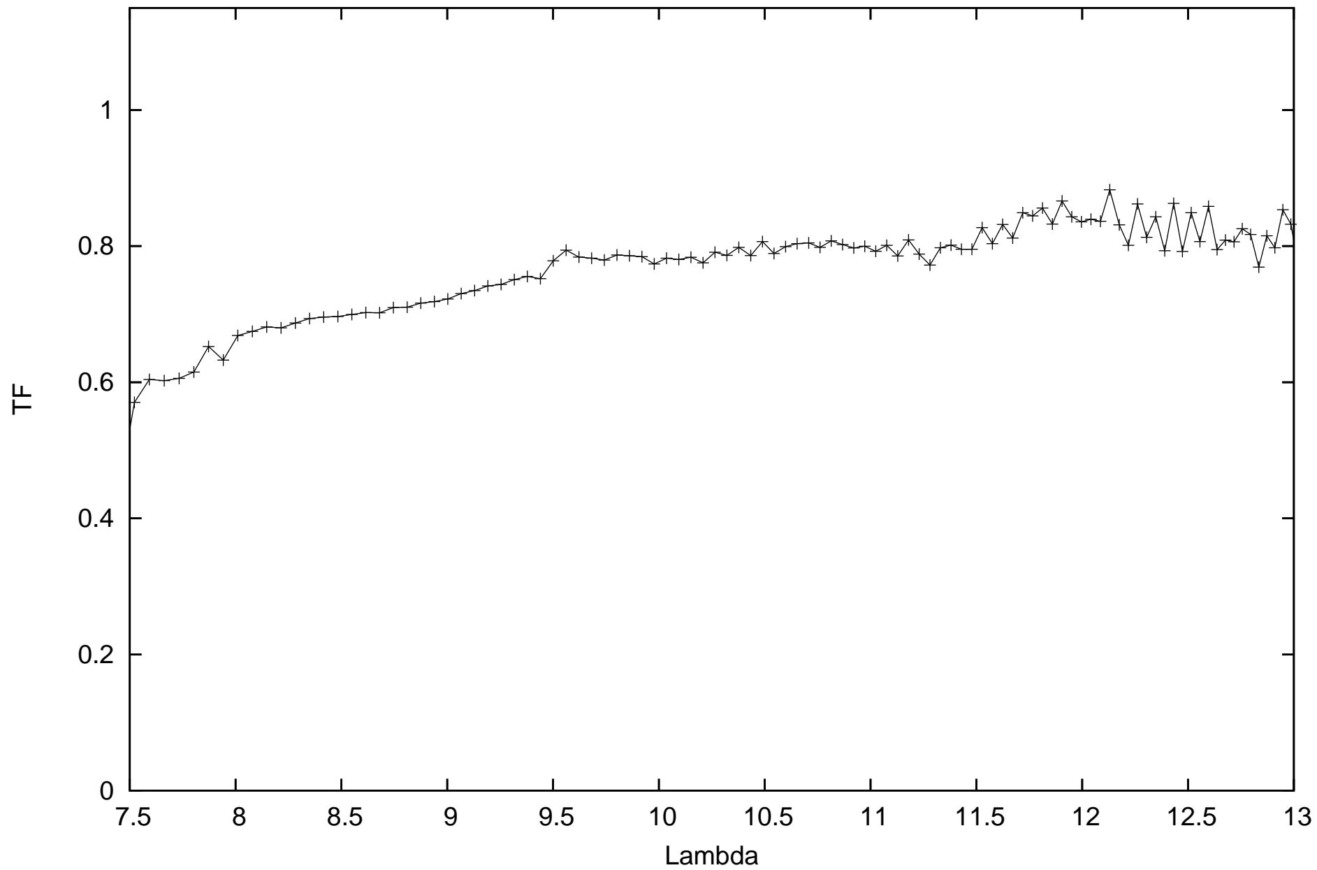
calHD81797_flux-1.49_diam9.14_r.MIDI.2014-02-03T04_37_21.000_D0H0
