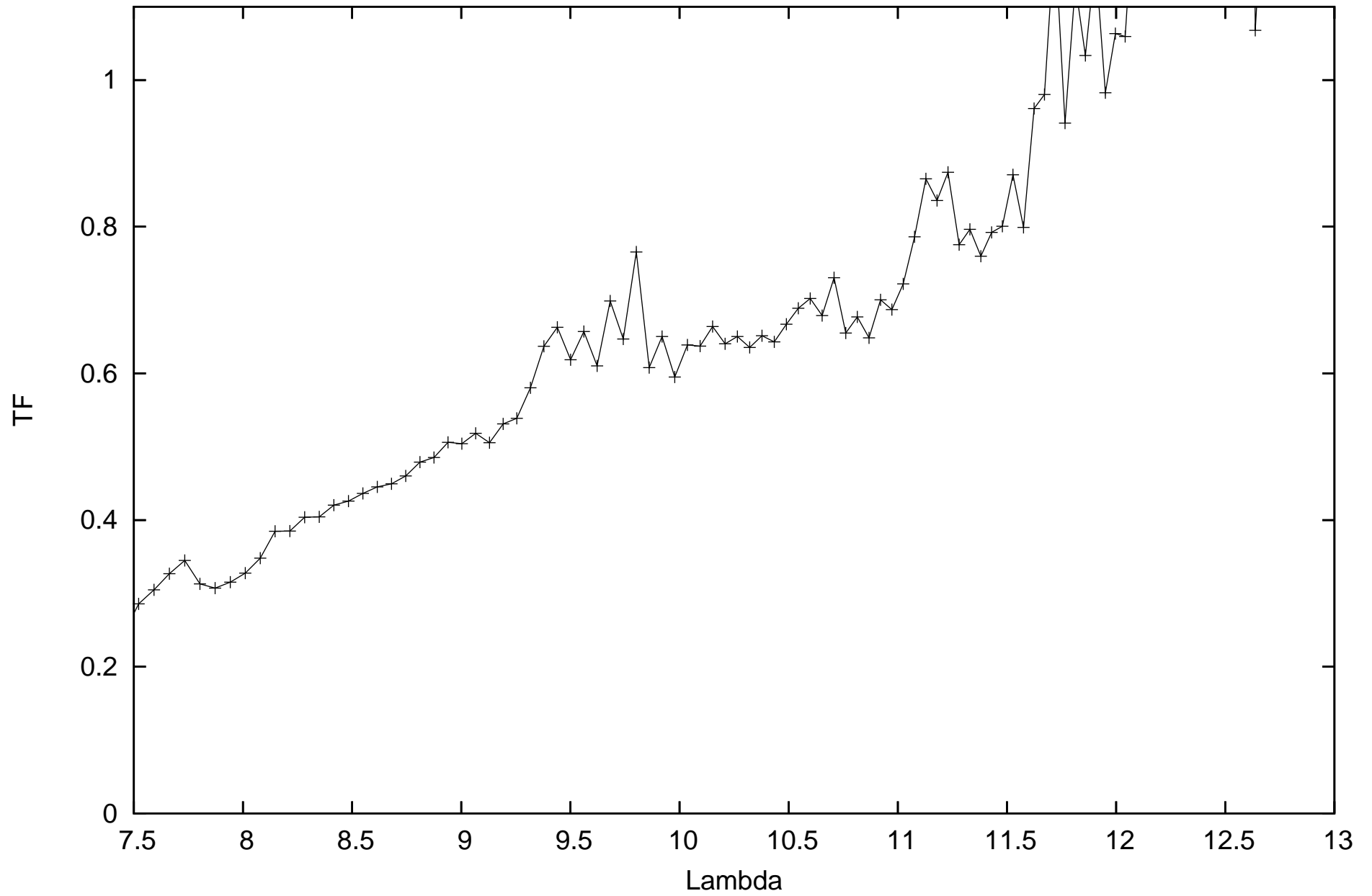
calHIP84969_flux1.79747_diam2._r.MIDI.2013-06-22T02_19_52.000_U3U4
