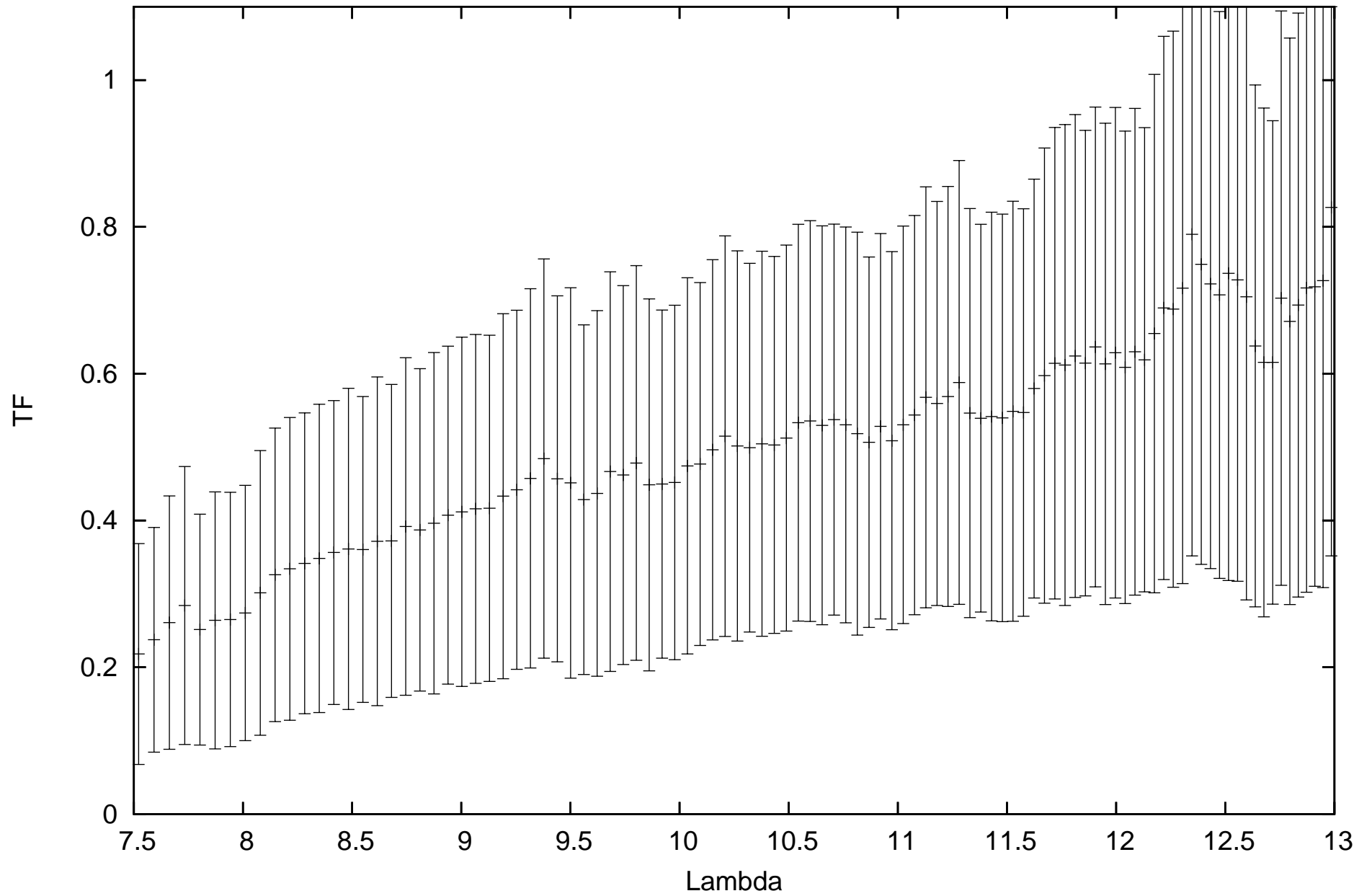
calHIP84969_flux1.79747_diam2._r.MIDI.2013-06-21T01_31_15.000_U1U4
