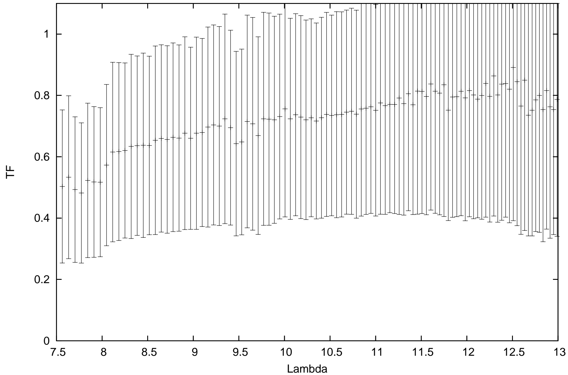
calHIP112748_flux1.25758_diam2.46_r.MIDI.2013-10-23T23_50_25.135_U2U3
