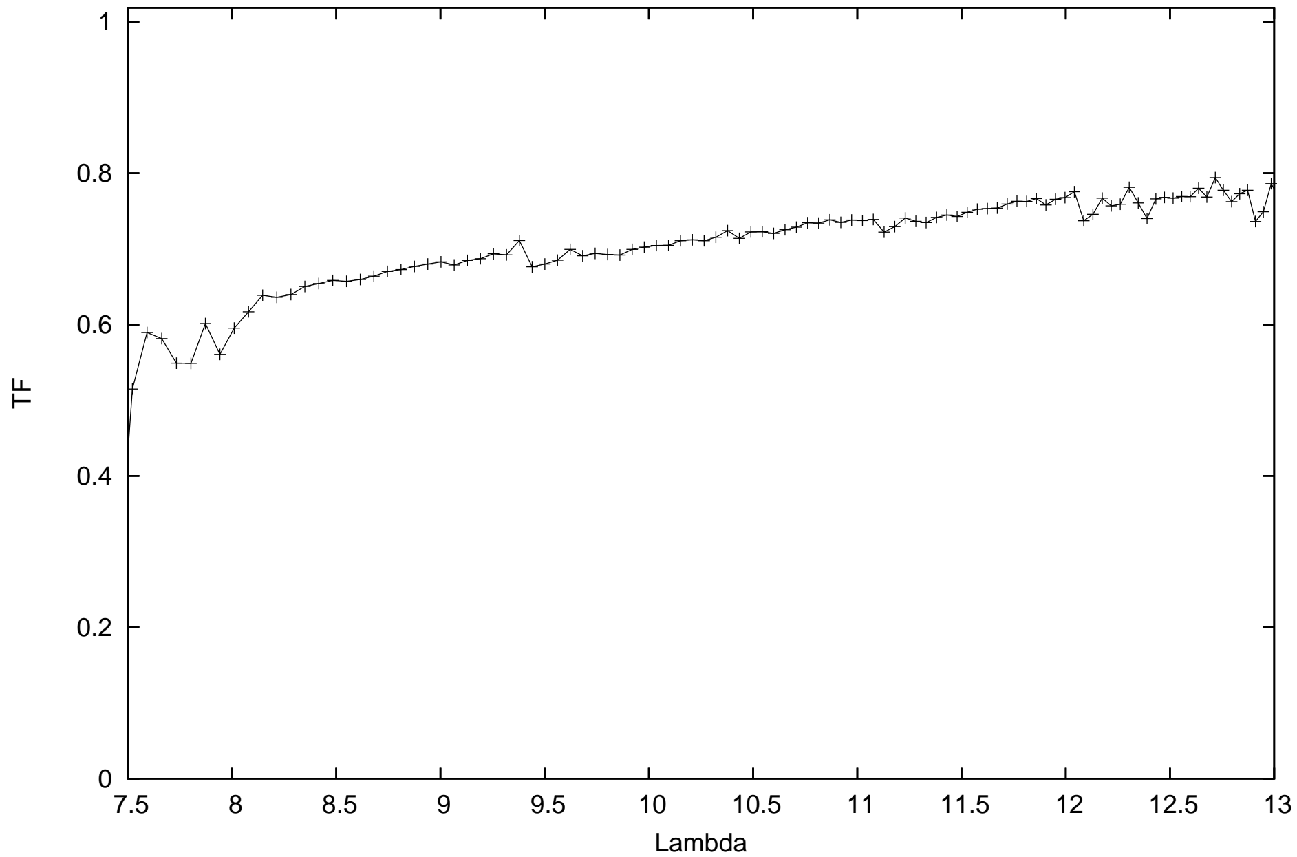
calHD98292_flux0.92_diam3.35_r.MIDI.2013-03-03T05_41_19.000_U2U4
