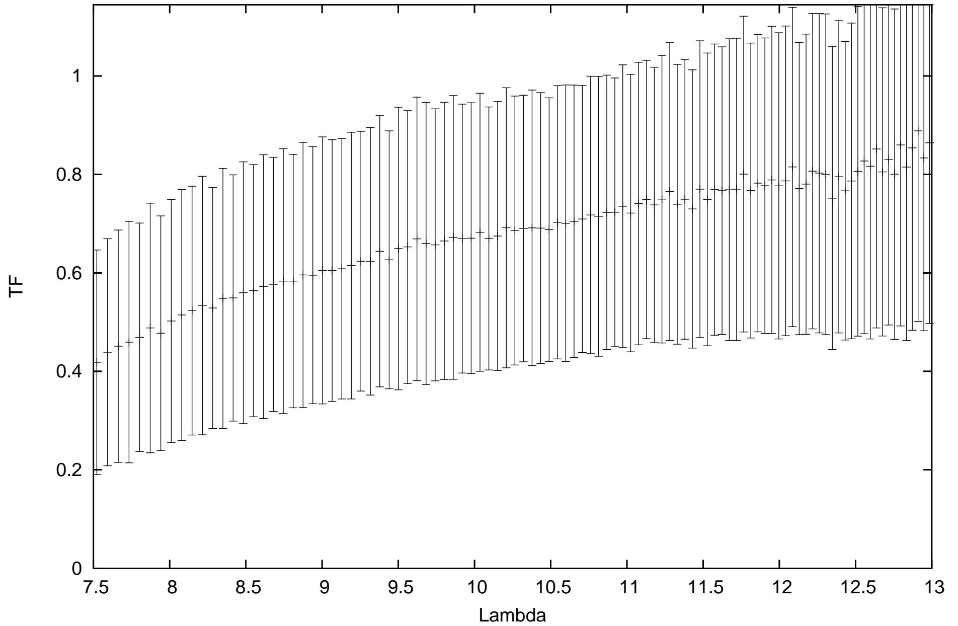
calHD167618_flux-1.82_diam11.66_r.MIDI.2013-08-21T01_27_28.000_G111
