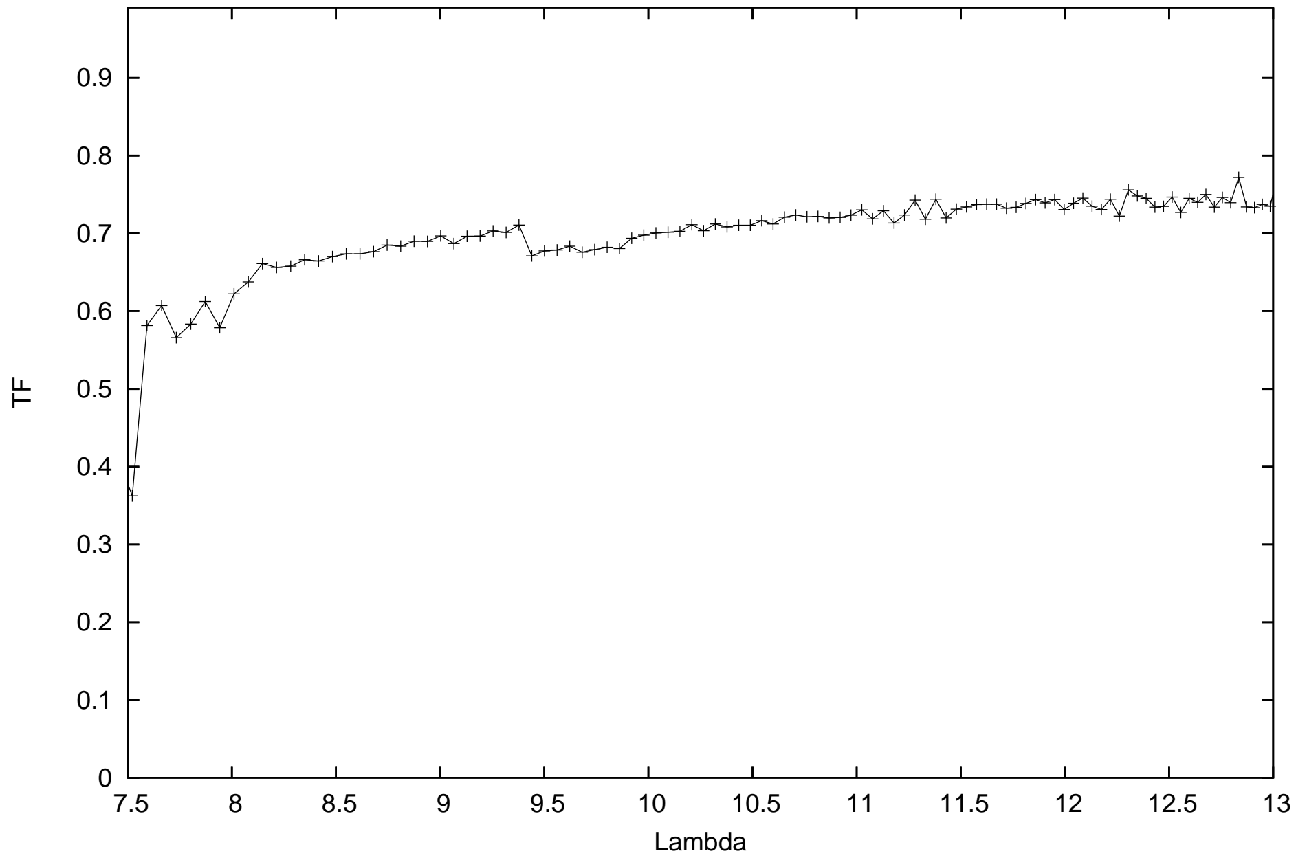
calHD102839_flux1.69_diam2.03_r.MIDI.2013-03-01T06_49_13.000_U3U4
