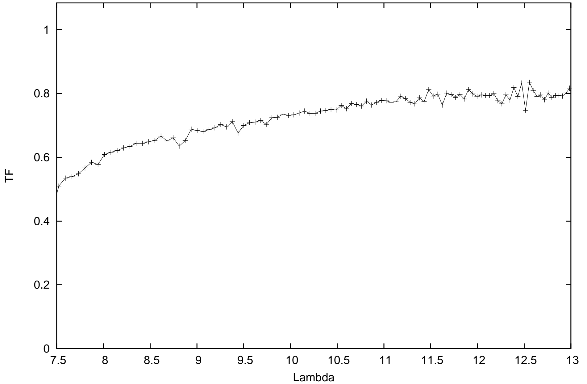
calHD167618_flux-1.82_diam11.66_r.MIDI.2013-07-29T01_55_31.000_G111
