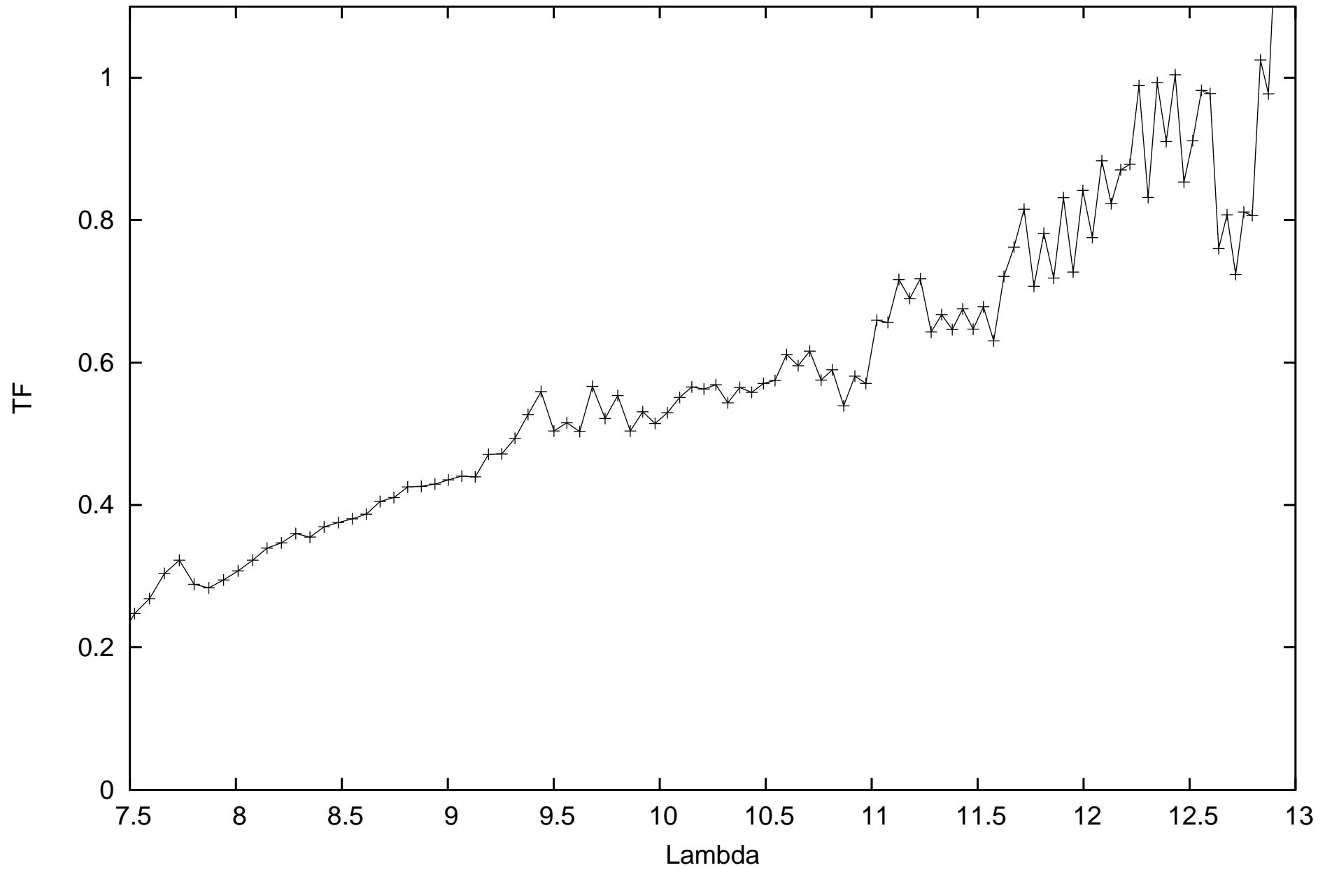
calHIP84969_flux1.79747_diam2._r.MIDI.2013-06-22T02_00_09.000_U3U4
