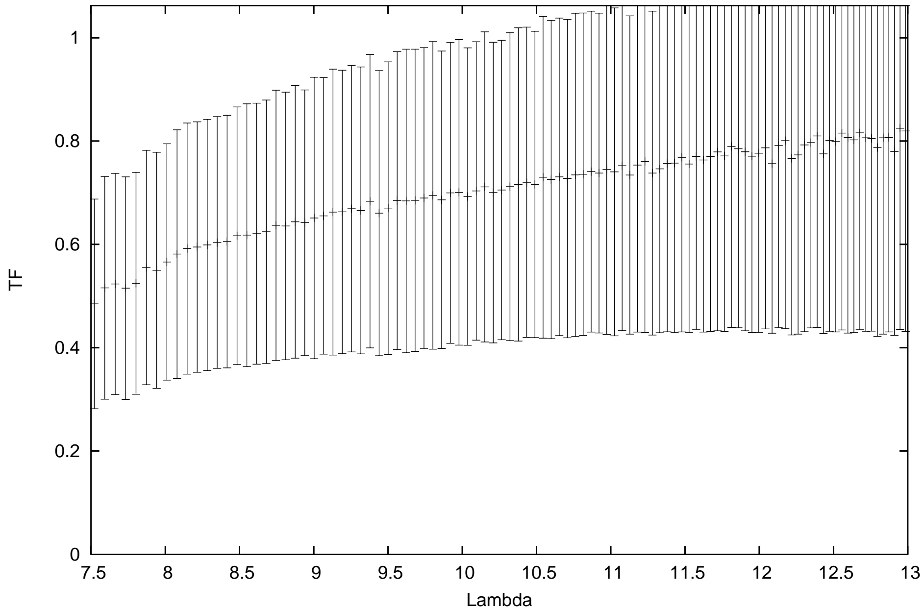
calHIP63066_flux1.00467_diam3.16_r.MIDI.2013-05-01T01_10_18.000_U1U4
