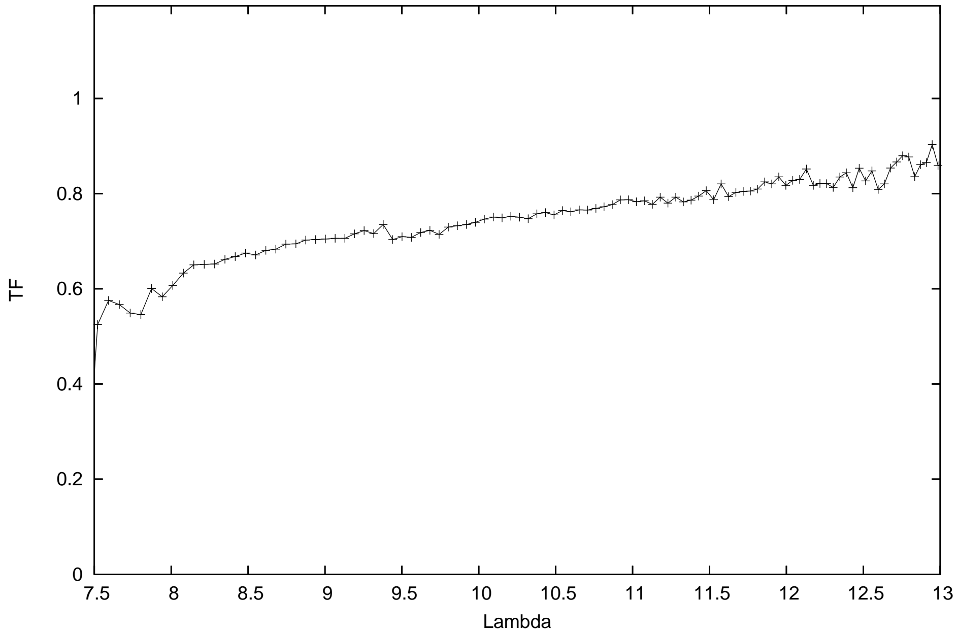
calHD98292_flux0.92_diam3.35_r.MIDI.2013-03-03T02_58_09.000_U2U4
