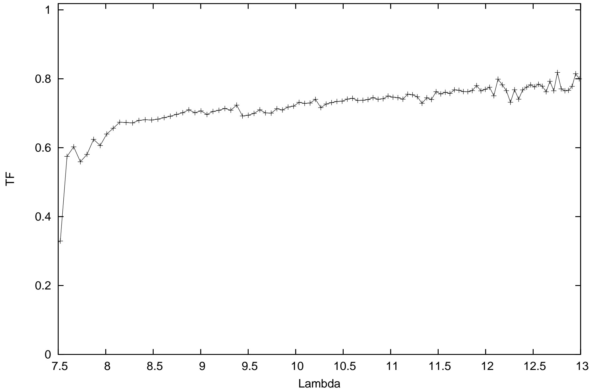
calHD102839_flux1.69_diam2.03_r.MIDI.2013-03-03T06_23_43.000_U2U4
