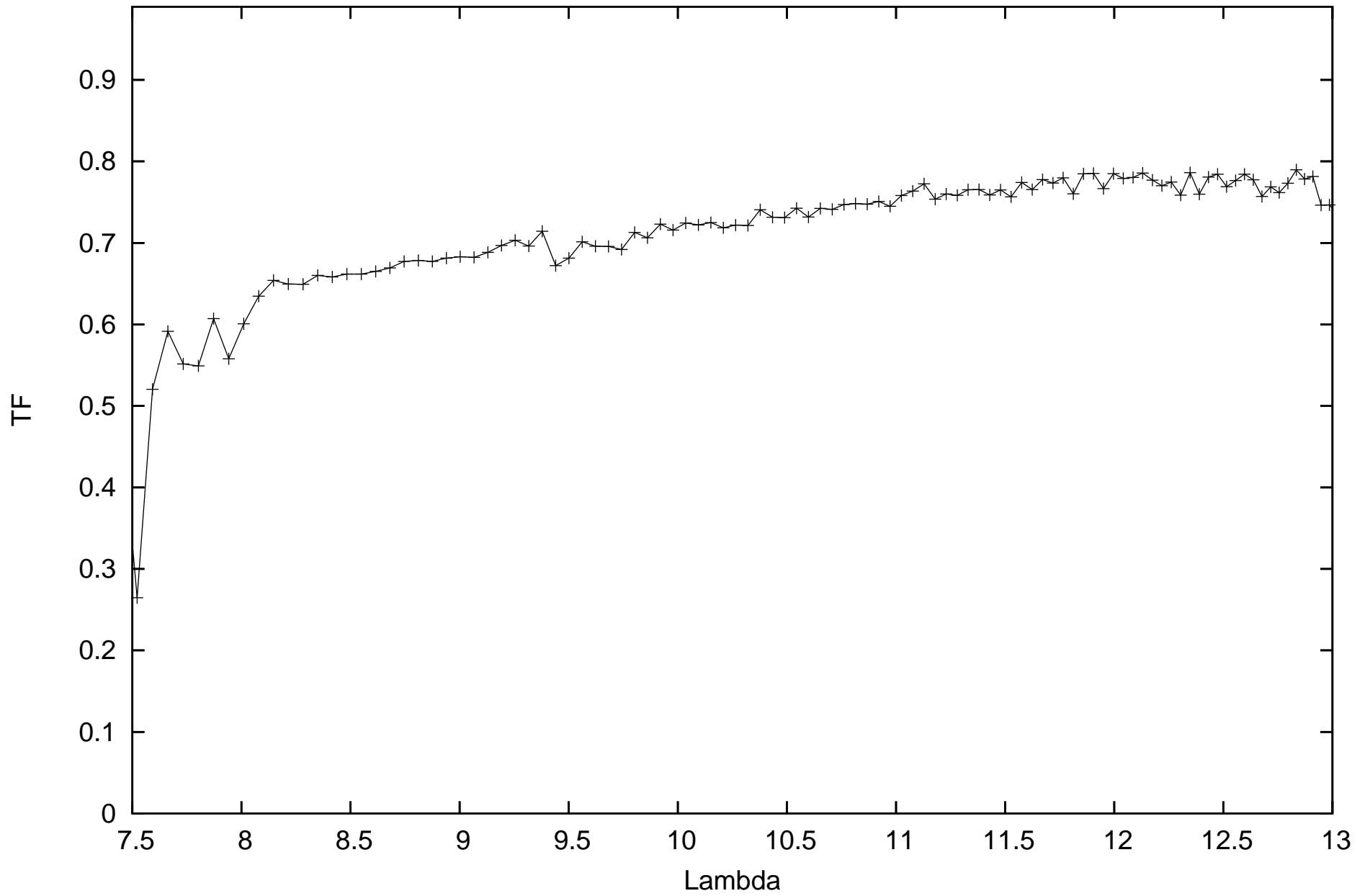
calHD102839_flux1.69_diam2.03_r.MIDI.2013-03-01T07_57_18.000_U3U4
