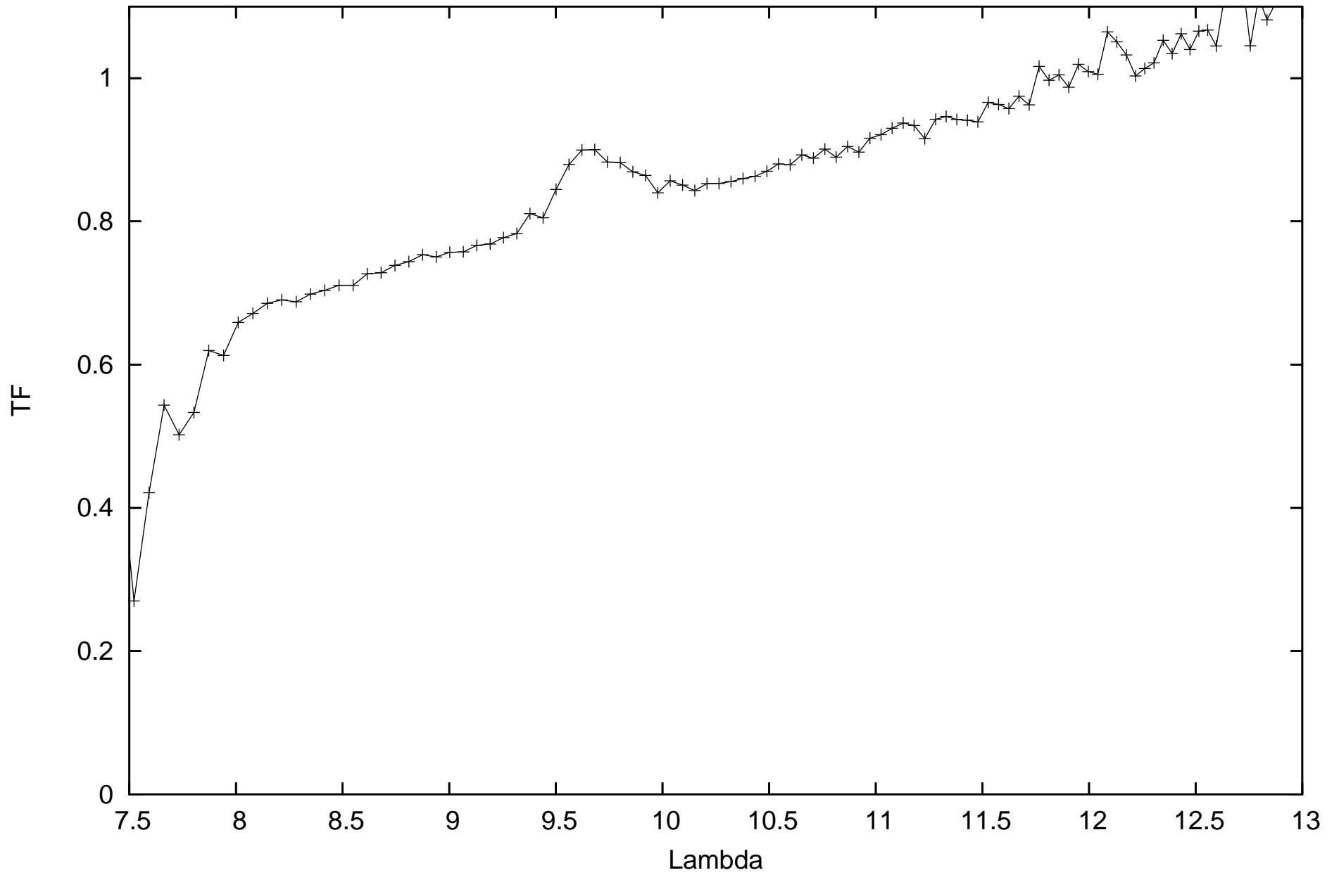
calHD102839_flux1.69_diam2.03_r.MIDI.2013-03-01T04_48_41.000_U1U4
