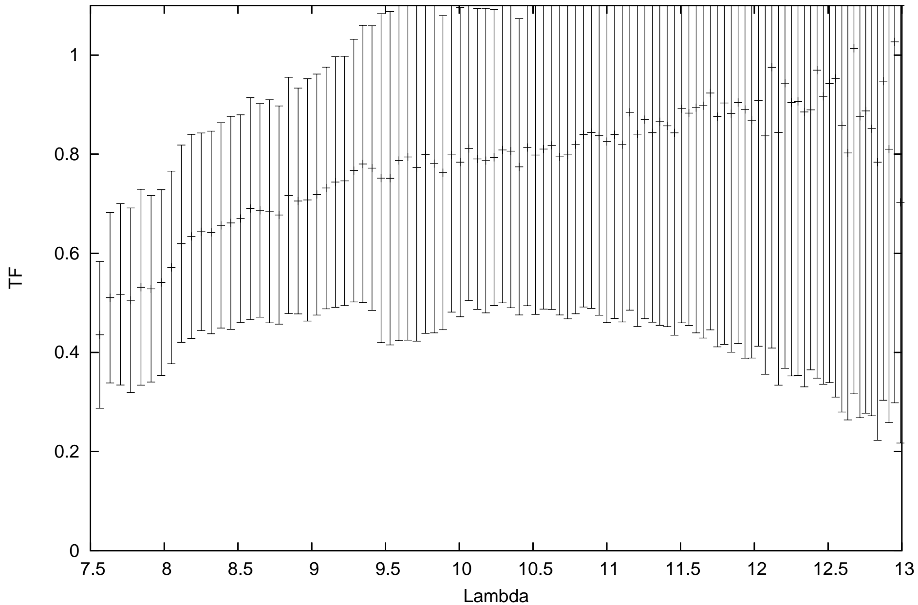
calHD167618_flux-1.82_diam11.66_r.MIDI.2012-07-22T01_46_46.112_B2A1
