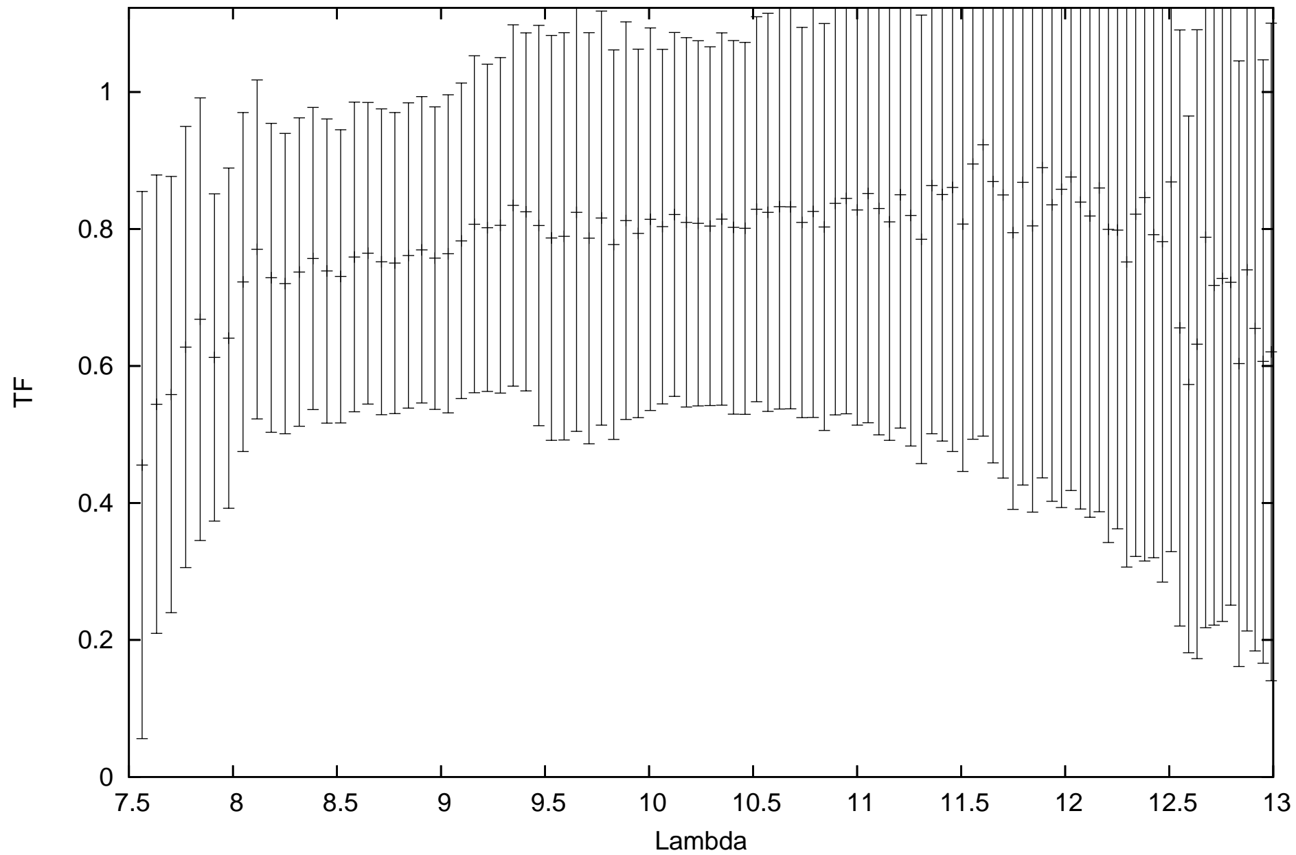
calHD81797_flux-1.49_diam9.14_r.MIDI.2012-02-01T04_41_59.135_B2A1
