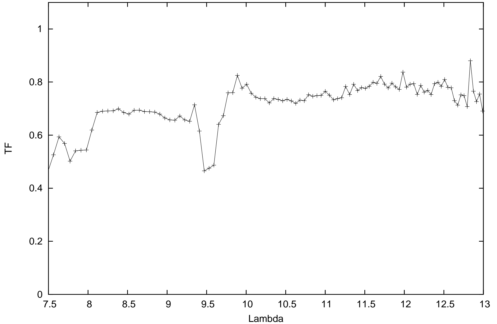
calHD167618_flux-1.82_diam11.66_r.MIDI.2011-11-04T00_26_57.293_G111
