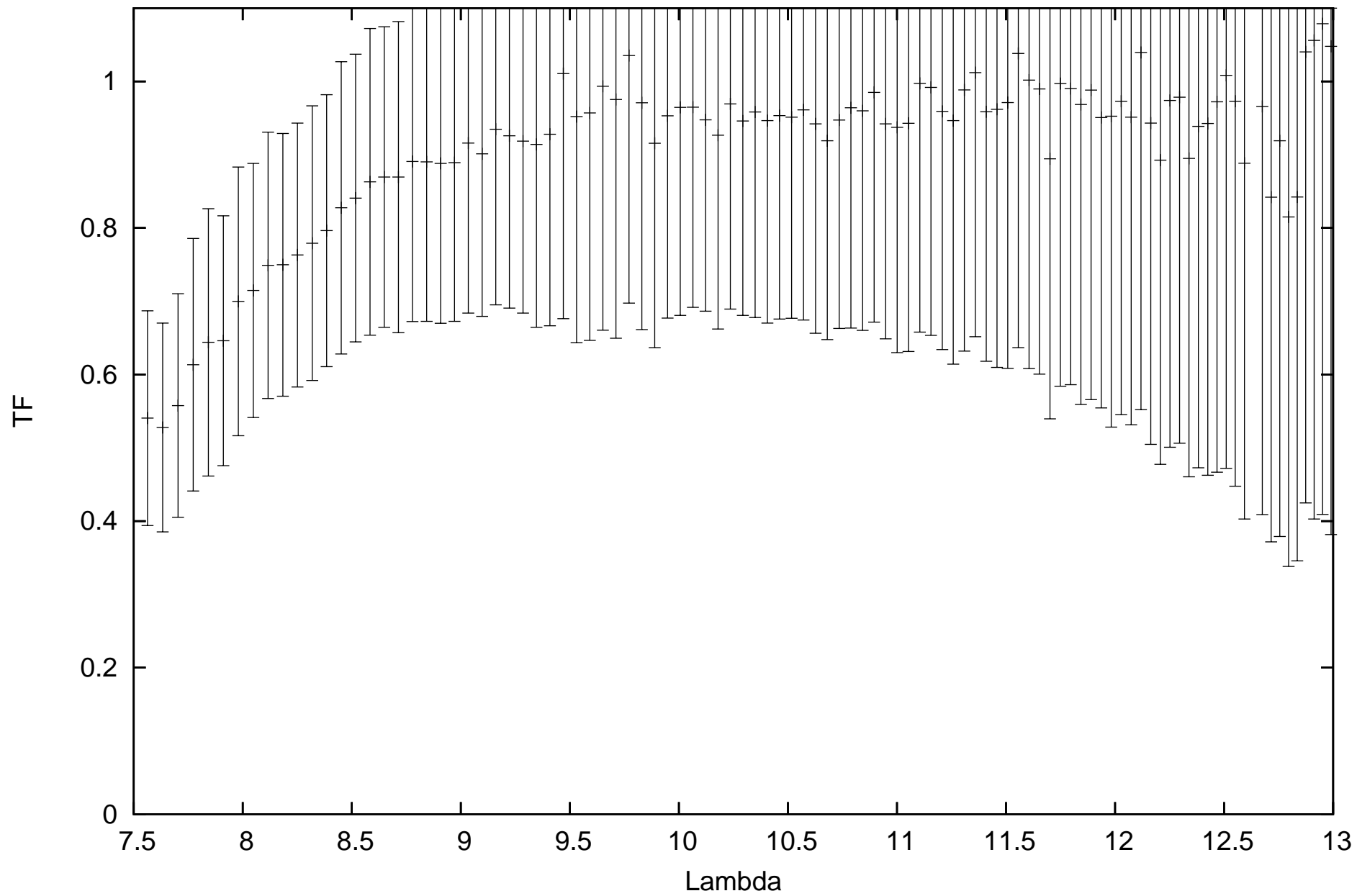
calHD167618_flux-1.82_diam11.66_r.MIDI.2011-06-11T08_20_04.179_B2A1
