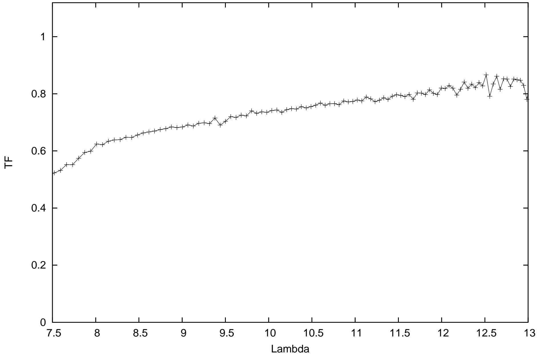
calHD167618_flux-1.82_diam11.66_r.MIDI.2010-08-22T02_10_40.000_H0I1
