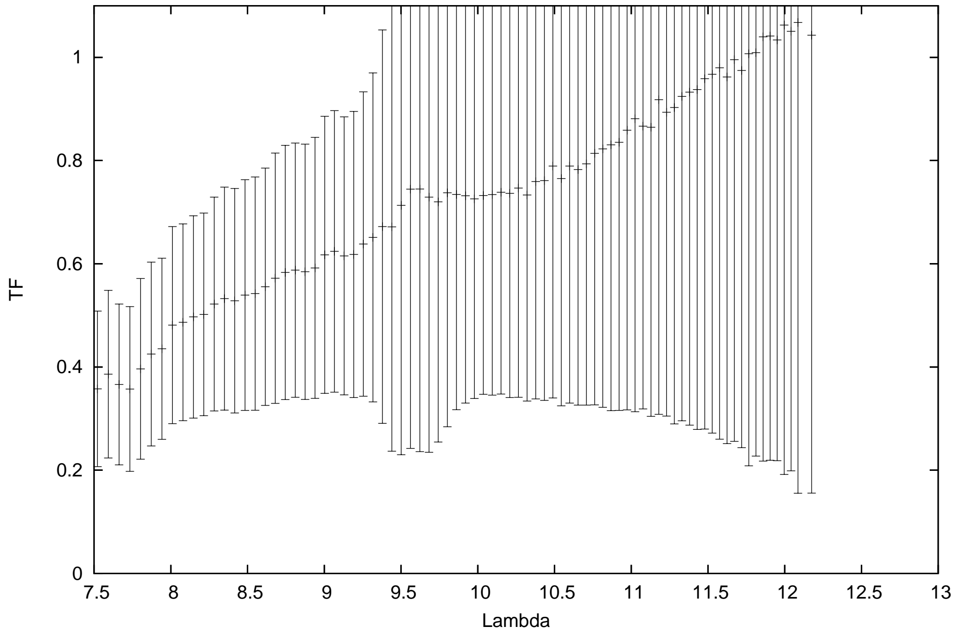
calHD023319_flux1.78_diam1.94_r.MIDI.2010-01-03T05_38_51.000_U3U4
