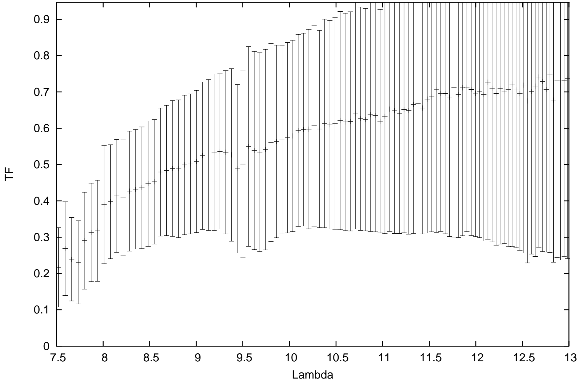
calHD023319_flux1.78_diam1.94_r.MIDI.2010-01-02T02_41_01.000_U1U3
