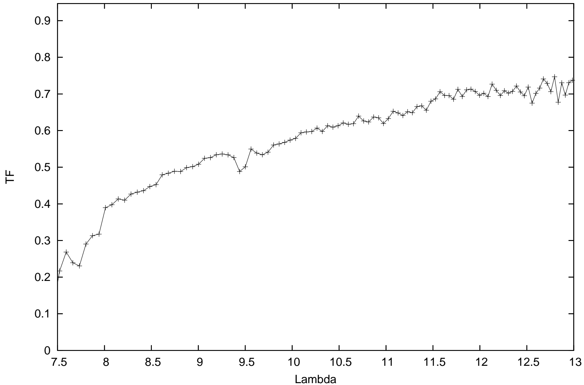
calHD023319_flux1.78_diam1.94_r.MIDI.2010-01-02T02_41_01.000_U1U3
